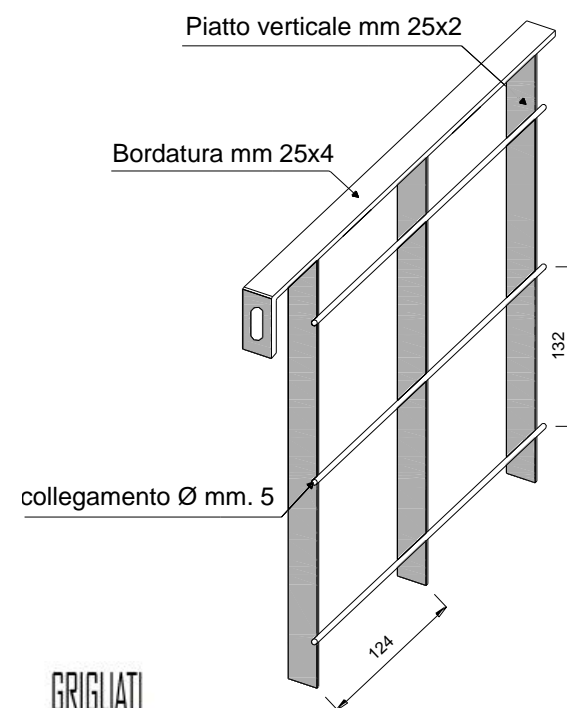
Recinzione modulare in grigliato elettrosaldato a maglia quadrata
